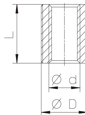
втулка с резьбой
